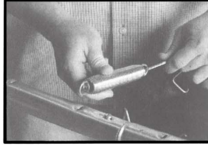
9 Присоедините пружину к кольцу на раме. Предупреждение: потребуется большое усилие, чтобы присоединить пружину к раме. Будьте осторожны и не защемите пальцы, можно получить серьезную травму!
