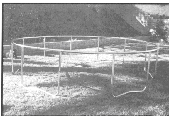
6 Присоедините собранные ноги.
