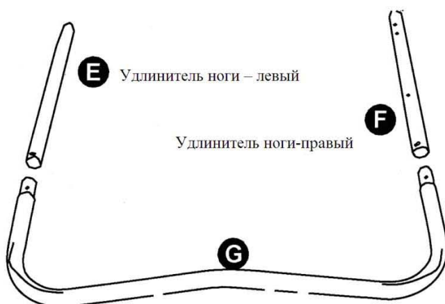
W-образная нога
