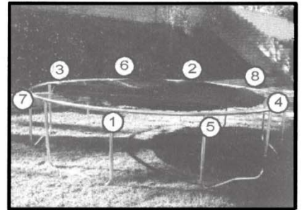
13 Повторите процесс размещения пружин на середине расстояния между уже установленными пружинами. Чтобы уравновесить натяжение пружины, присоедините противоположный конец предыдущей пружины.
